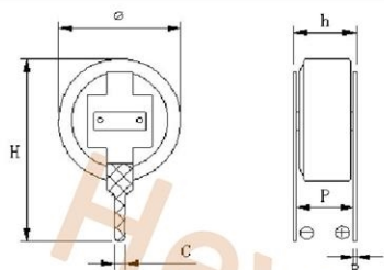
V型
