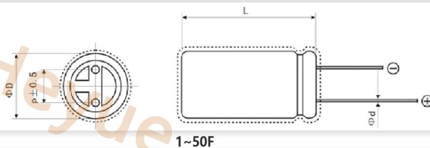
产品图纸
